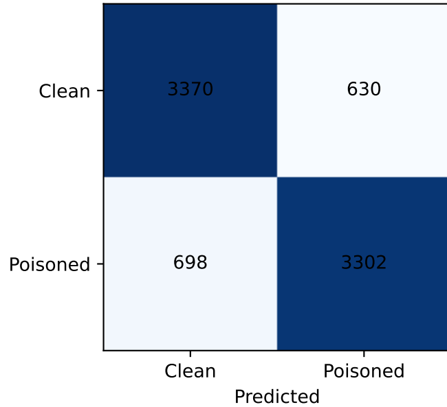
SVM
