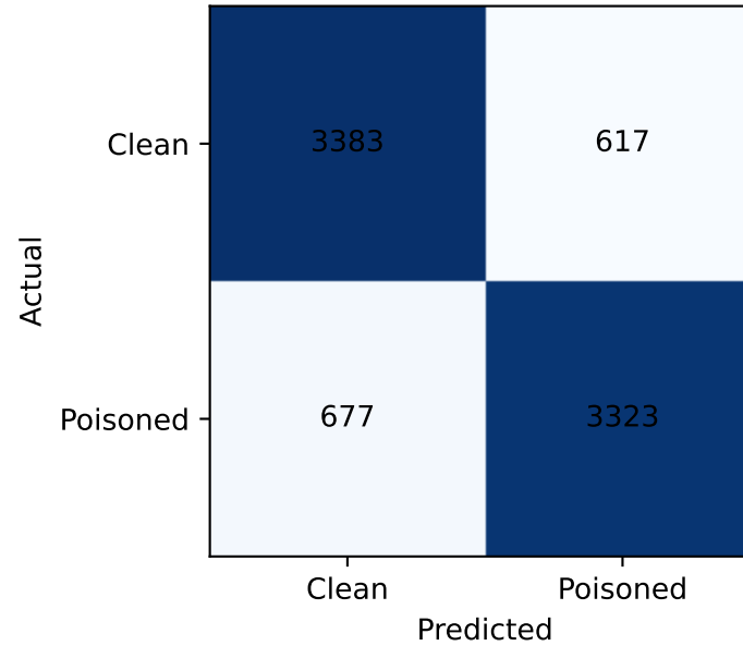
KNN
